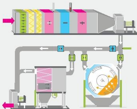
Обработка воздуха с конденсатоотводом для дражирования сахаром
