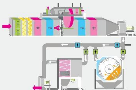
Обработка воздуха с осушением для дражирования сахаром и сахарозаменителем
